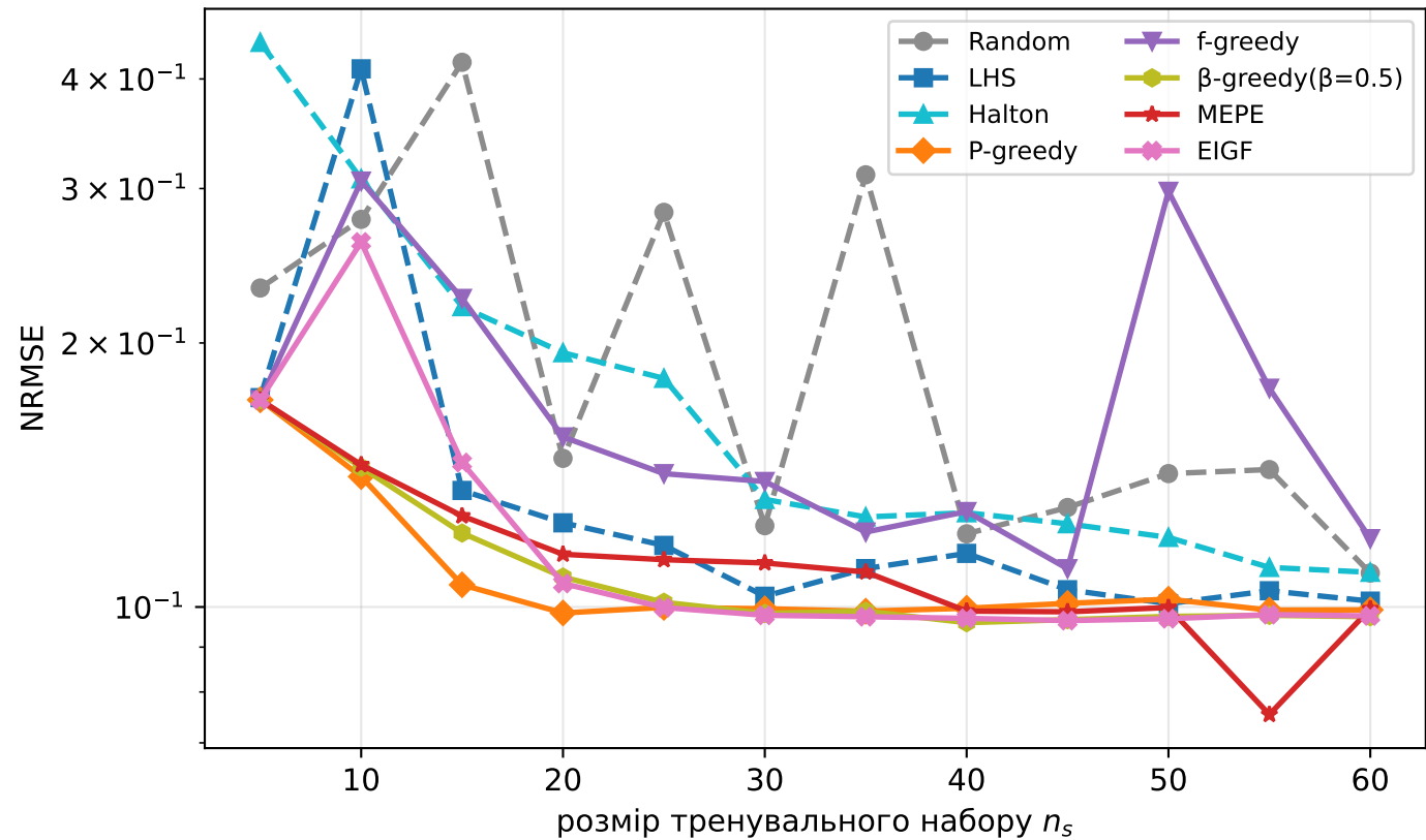
Збіжність помилки сурогата для J_2
